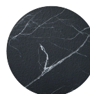
CALCATA
