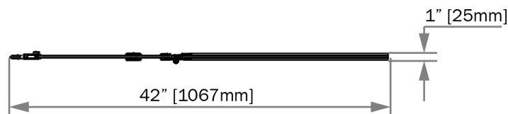
TOP VIEW - VUE DE DESSUS
